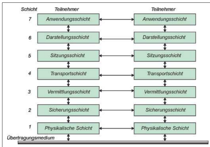
Bild 12: Das TCP/IP-Protokoll fasst einige Schichten des ISO/OSI-Modells zusammen.
