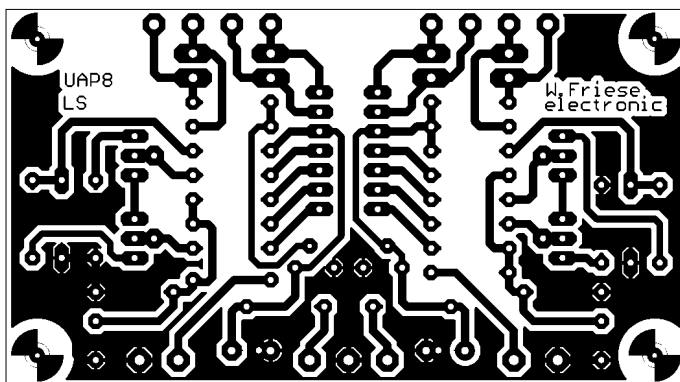
Bild 95: Leiterseite der Platine UAP8 im Maßstab 1:1
