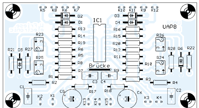
Bild 96: Bestückungsplan der einseitigen Platine UAP8
