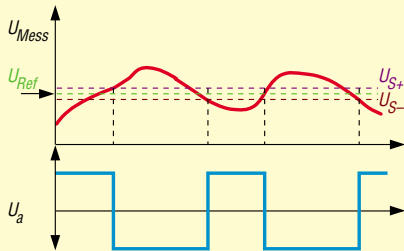
Bild 87: Ausgangsspannung des Komparators mit Hysterese (Bild 86) in Abhängigkeit des Messsignals. Durch die Hysterese liegt der Einschaltpunkt (gemeint ist hier das Durchschalten des Ausgangs auf -U S ) oberhalb der Referenzspannung und der Ausschaltpunkt etwas unterhalb des Referenzpunkts.
