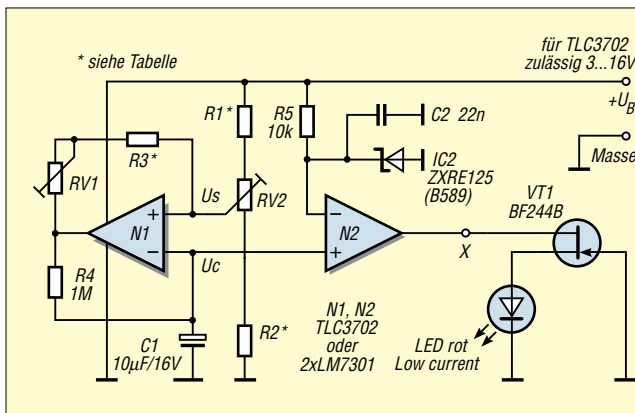
Bild 1: Für die Schaltung als Teil eines Gesamtgeräts ist keine Platine erforderlich. Die OPVs arbeiten mit nur einer Spannungsquelle.
