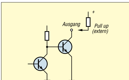
Bild 88: Die speziellen integrierten Komparatorbausteine werden sehr häufig mit offenem Kollektor des Ausgangstransistors angeboten, an den dann ein externer Pull-Up-Widerstand geschaltet wird.
