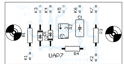
Bild 99: Bestückungsplan der einseitigen Platine UAP 7
