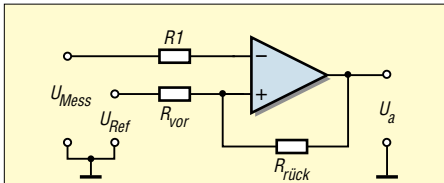
Bild 86: Komparator für Spannungen gleicher Polarität mit Hysterese (verursacht durch Einfügen des Rückführwiderstands R rück )
