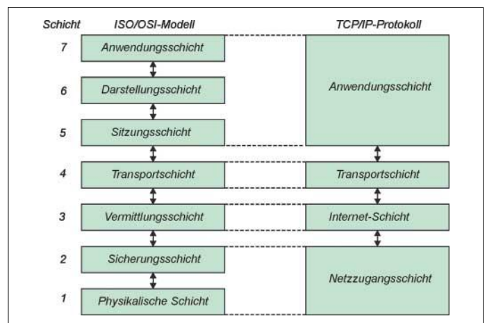
Bild 11: Das ISO/OSI-Referenzmodell ist die Grundlage aller Datenübertragungen.
