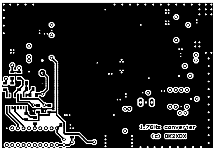
Bild 11: Unterseite der zweiseitigen Platine; fast die gesamte Kupferbeschichtung dient als Massefläche.
