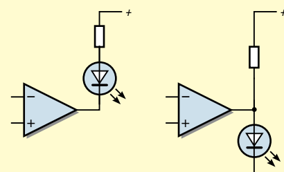
Bild 90: Zwei unterschiedliche Methoden, eine LED durch einen Komparator mit offenem Kollektor des Ausgangstransistors anzusteuern. Die LED leuchten jeweils bei inversen Schaltzuständen des Komparators.
