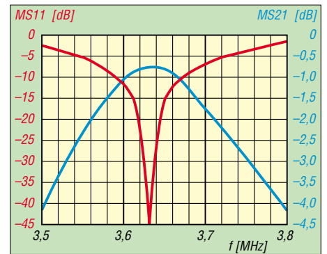
Bild 15: Anpassung (rot) und Amplitudengang (blau) des T-Glieds inkl. RG58-Leitung
