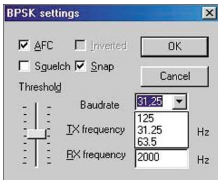
Bild 1: Einstellung der digitalen Betriebsarten BPSK63 bzw. BPSK125 im Untermenü der BPSK31-Einstellung
