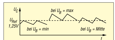
Bild 3: Spannung am Kondensator C1 bei verschiedenen Werten von U_B
