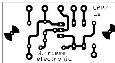
Bild 98: Leiterseite der Platine UAP 7 im Maßstab 1:1
