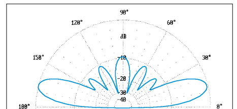
Bild 5: Flache Abstrahlung im 10-m-Band bei der gestreckten Ausführung; hier in Hauptstrahlrichtung 57°/237°; Außenring 11,42 dBi
