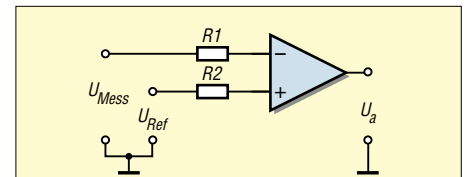
Bild 83: Einfacher Komparator für Spannungen ( U_{\text{Mess}} , U_{\text{Ref}} ) mit gleicher Polarität
