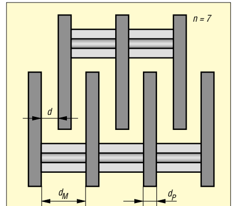
Bild 4: Aus der Dicke der verwendeten Zwischenstücke und des Bleches ergibt sich der Plattenabstand.
