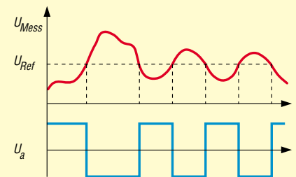
Bild 84: Die Ausgangsspannung des Komparators im Bild 83 in Abhängigkeit der angelegten Messspannung. Das Ausgangssignal nimmt nur die beiden Zustände „positive Sättigungsspannung“ bzw. „negative Sättigungsspannung“ an.
