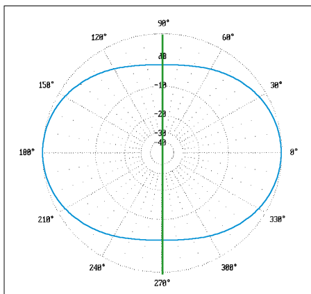
Bild 2: Im 40-m-Band weist die Antenne nahezu Rundstrahlverhalten auf; hier bei 45° Erhebungswinkel, Außenring 7,28 dBi
