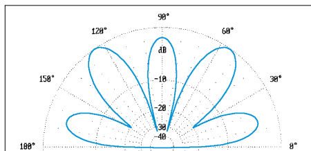
Bild 6: Erhebliche Steilstrahlung im 10-m-Band bei der Inverted Vee, hier in Hauptstrahlrichtung 59°/239°; Außenring 8,26 dBi.
