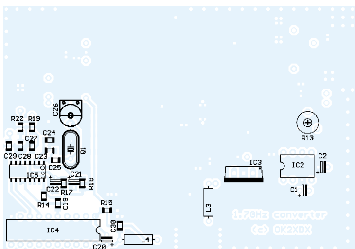
Bild 12: Bestückung auf der Platinenunterseite mit dem Digitalteil; mehr Bauelemente sind für die Steuerung nicht erforderlich.
