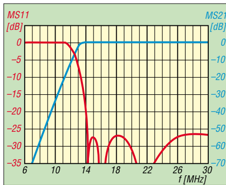
Bild 13: Anpassung (rot) und Amplitudengang (blau) des 13,9-MHz-Hochpasses
