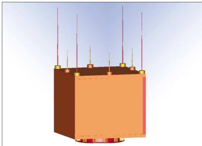
Die Form von VUSat mit den VHF/UHF-Antennen. Der Start erfolgt voraussichtlich am 10.10.03 in einen 817 km hohen, zirkularen Orbit. Die Inklination beträgt 98,68° und die Exzentrizität 0,002°. Ein Orbit dauert etwa 7100 s. Grafik: AMSAT
