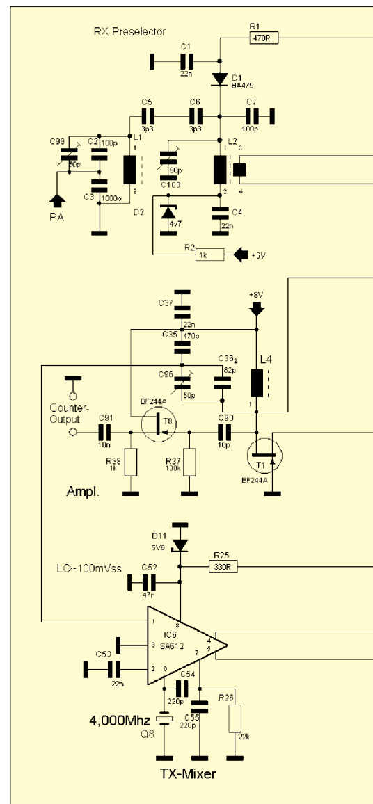
Bild 1: Da sich fast die gesamte Schaltung auf einer einzigen Leiterplatte befindet, muss man bei der Endmontage „nur“ die Bedienelemente und Buchsen mit Grundplatine und DDS-VFO verbinden.
