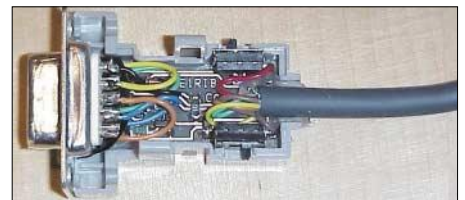
Bild 5: Ansicht der Platine im Steckergehäuse
