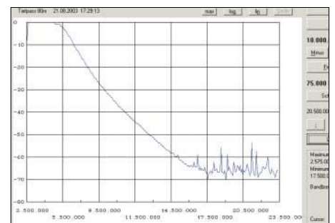
Bild 2: Frequenzgang des 40-m-Tiefpassfilters, aufgenommen mit dem NWT [2]
