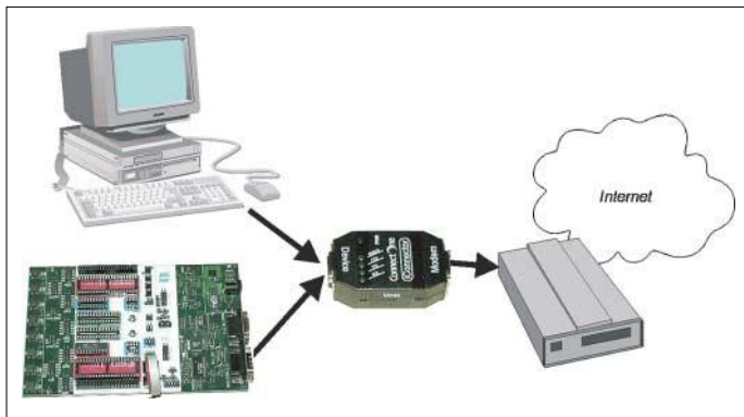
Bild 10: Den iConnector kann man als eine Ansteuermöglichkeit mit dem Starterkit STK500 für AVR-Controller verbinden.
