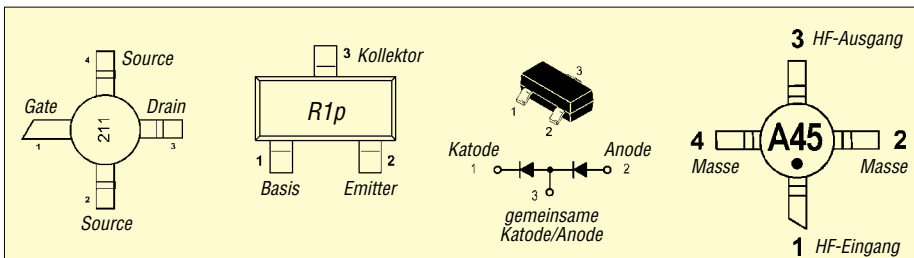
Bild 15: Für die Bauelemente sind verschiedene Typen verwendbar. Hier dargestellt sind die Anschlussbelegungen eines AFT21186, BFR93, MMD353 und SGA4586 (v.l.n.r.).
