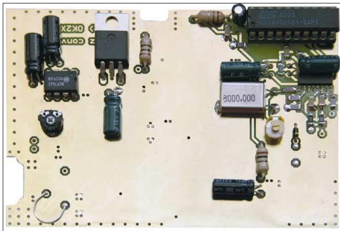
Bild 9: Die digitale Seite der bestückten Konverterplatine weist eine große Massefläche auf.
