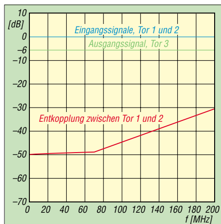
Bild 7: Frequenzgang von Durchgangsdämpfung und Entkopplung der Wheatstone-Messbrücke aus Bild 6
