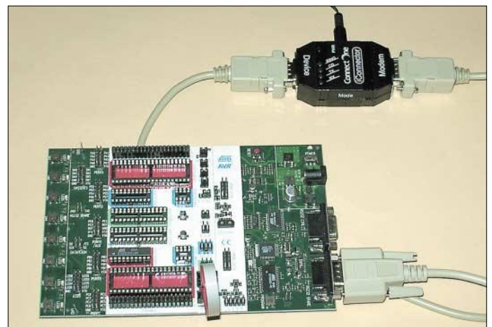
Bild 9: Eine Testkonfiguration ist mit dem STK500 oder einem PC und dem iConnector möglich.
