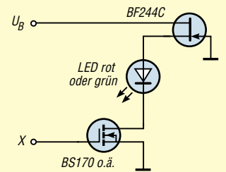
Bild 2: Die Hilfsschaltung zur Ansteuerung von LEDs mit größeren Strömen wird anstelle von VT1 mit dem Punkt X verbunden.
