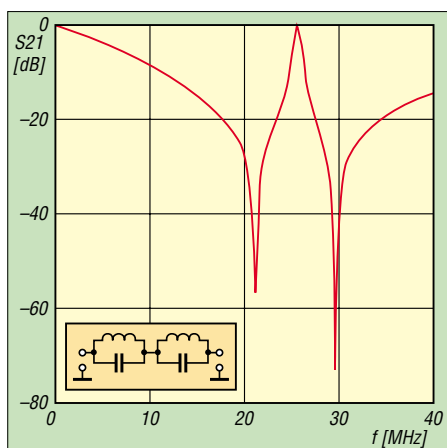
Bild 2: Simulierter Frequenzgang der Trapanordnung sowie Ersatzschaltbild
