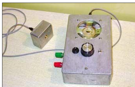
Empfänger: Der abgesetzte Laserdetektor (links) mit Anschlusskabel, das die empfangene NF mit dem Verstärker (rechts) verbindet auch der Spannungsversorgung des Detektors dient.
