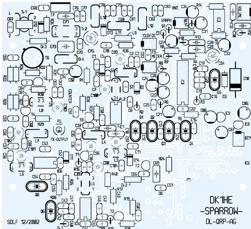
Bild 5: Trotz der relativ dichten Bestückung ist ein Aufbau durch die stufenweise Herangehensweise in kurzer Zeit realisierbar.
