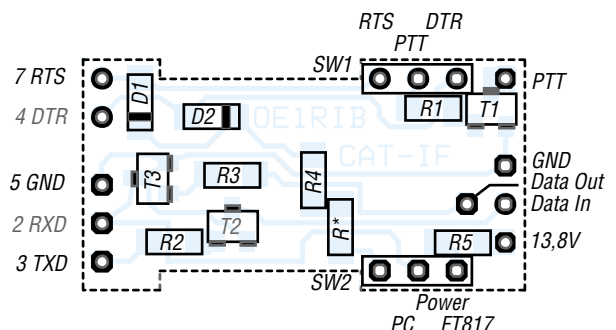
Bild 3: Die Bestückung der einseitigen Platine erfolgt auf der Leiterseite
