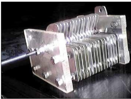
Bild 1: Die Endstücke aus Plexiglas erlauben die isolierte Montage des Drehkondensators.
