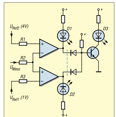
Bild 91: Fensterkomparator mit drei Anzeige-LED (realisierbar mit UAP8 und UAP11); Bedeutung der LED:
