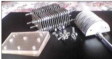
Bild 2: Den fertigen Drehkondensator kann man leicht wieder zerlegen und durch Änderung der Plattenzahl die Endkapazität beeinflussen.
