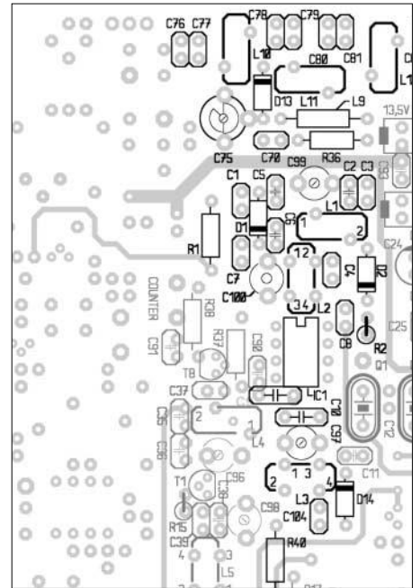
Bild 3: Der stufenweise Aufbau ist in der Bau-Mappe durch unterschiedlich gekennzeichnete Bauelemente sichtbar.
