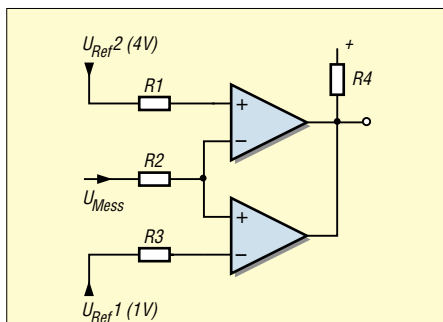
Bild 89: Ein Fensterkomparator – Komparatorausgänge können auch zusammengeschaltet werden und gemeinsam über einen Pull-up-Widerstand an Plus gelegt werden; eine Messspannung zwischen 1 V und 4 V ergibt am Ausgang High-Signal, eine über 4 V oder unter 1 V ein Low-Signal.
