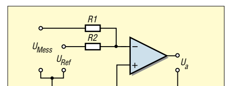
Bild 85: Einfacher Komparator für Spannungen ( U_{\text{Mess}} , U_{\text{Ref}} ) unterschiedlicher Polarität
