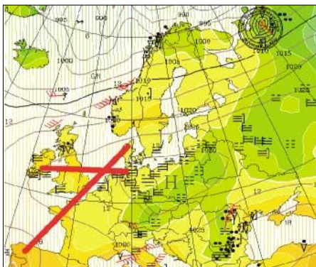
Isobaren und Temperaturen am 14.9. (Uni Köln)
