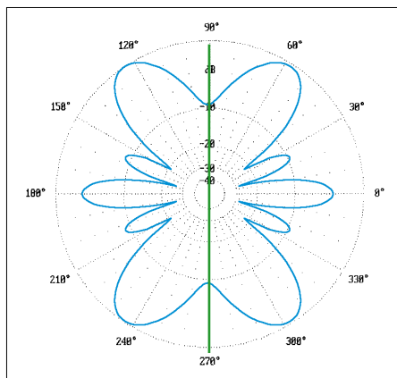
Bild 3: Aufspaltung des Azimutaldiagramms im 10-m-Band, hier bei 16° Erhebungswinkel, Außenring 11,42 dBi
